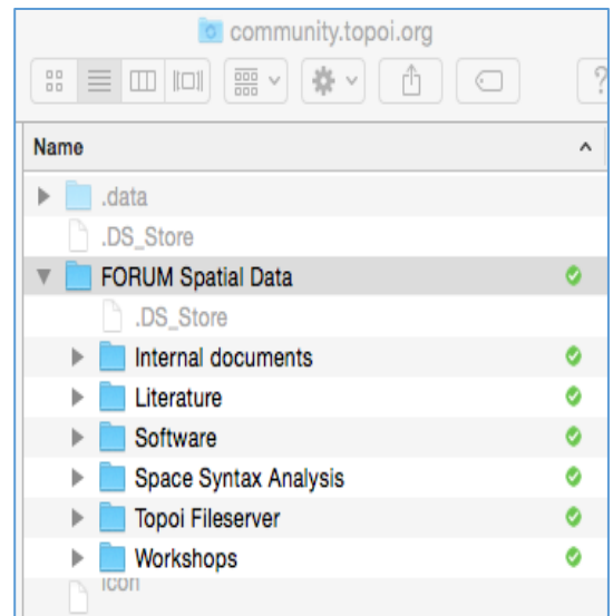
Abbildung 4: OS X
